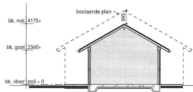
Doorsnede B-B schaal 1 : 100
